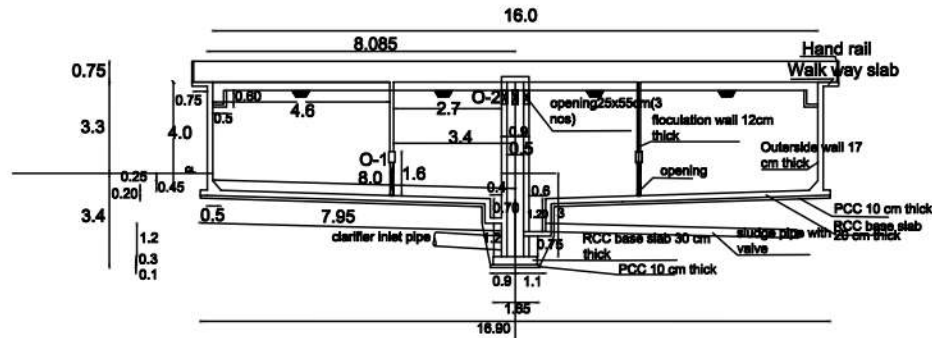
Clariflocculator
